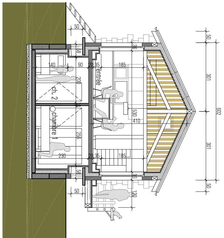
COUPE AA
