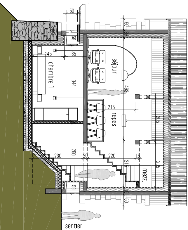
COUPE C-C
