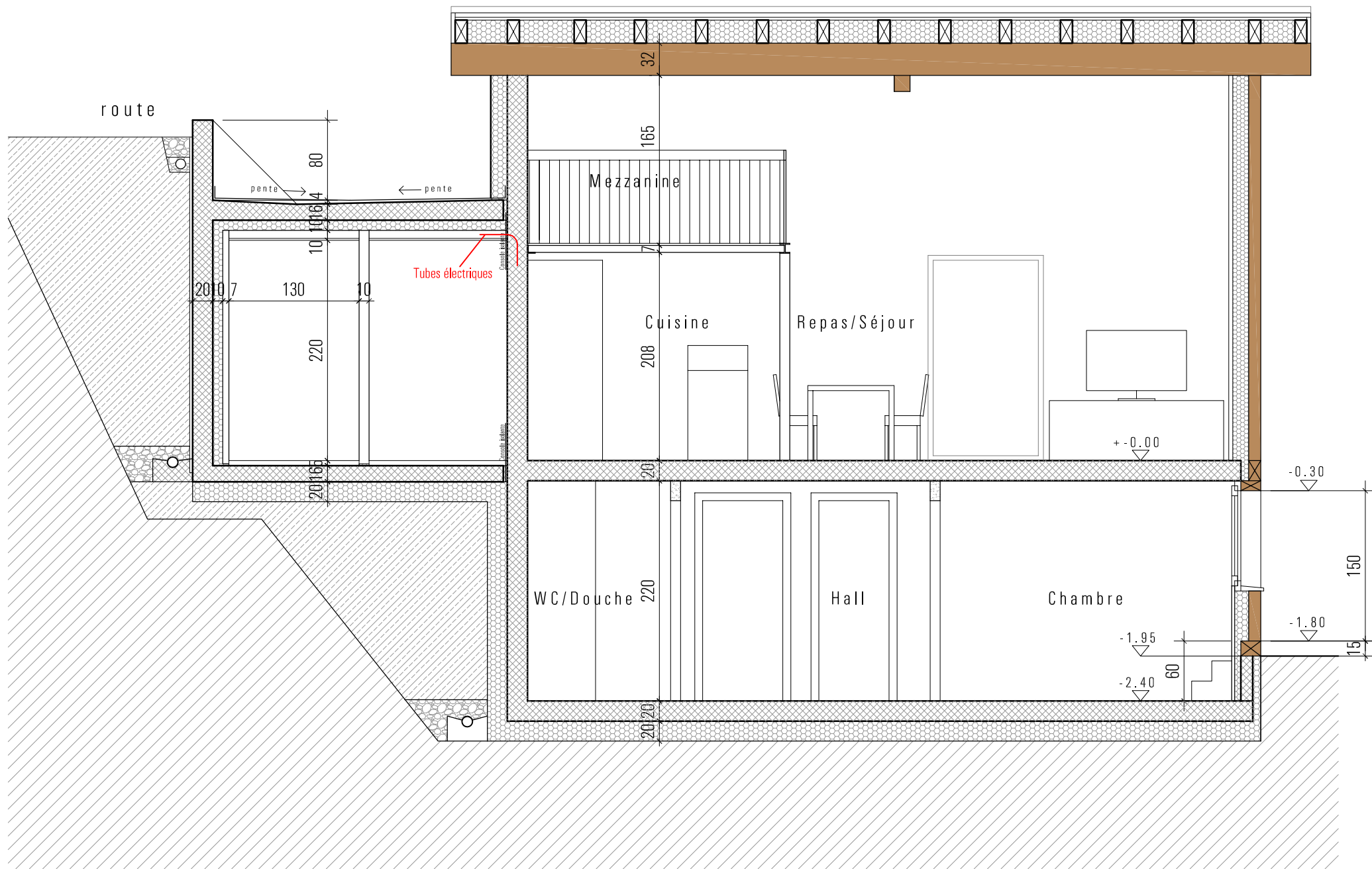
Coupe b-b
