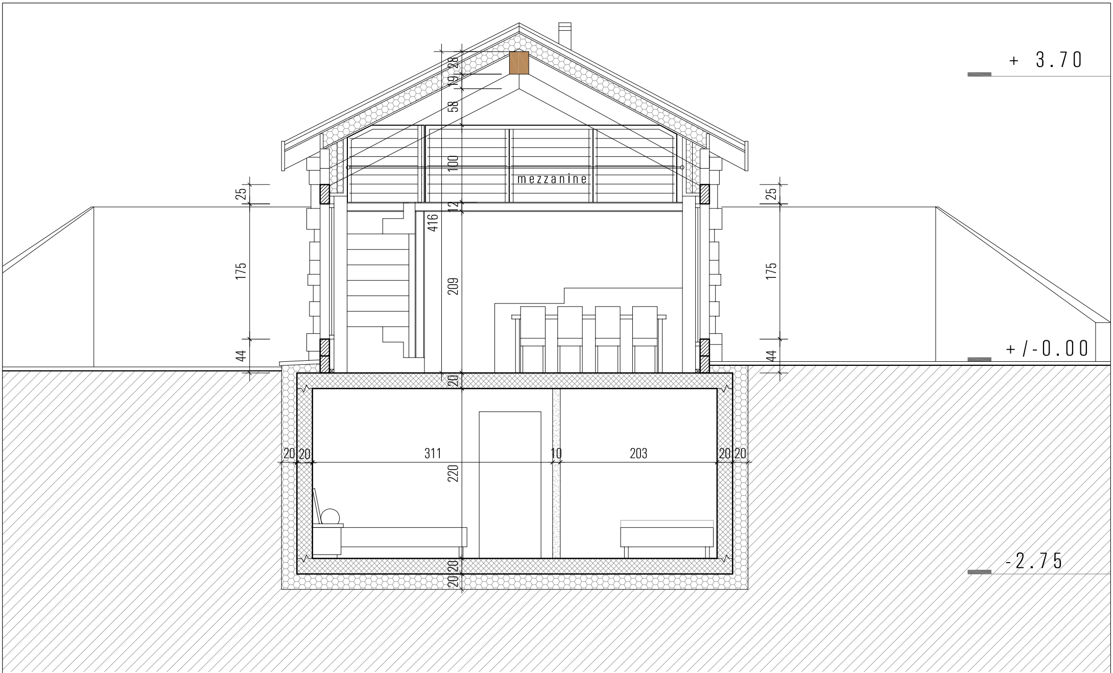
Coupe a-a
