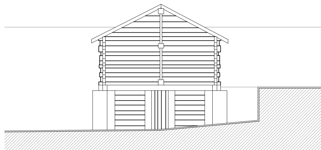
façade ouest
