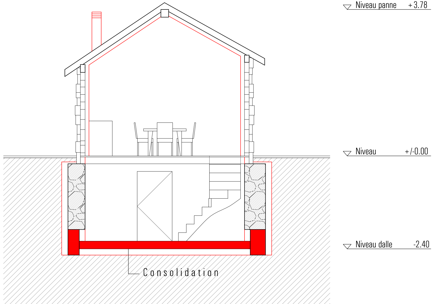
Coupe A-A
