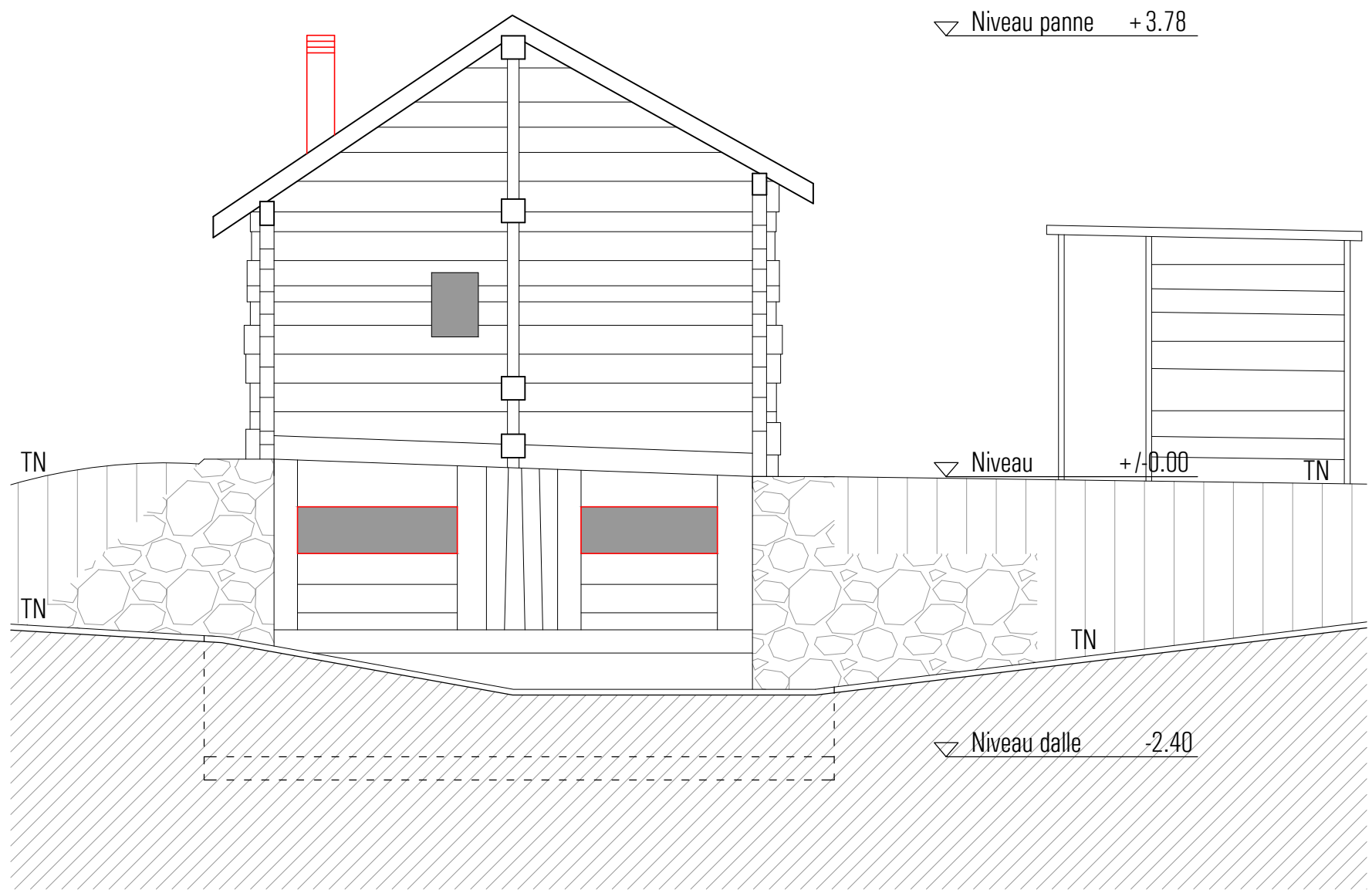
façade ouest
