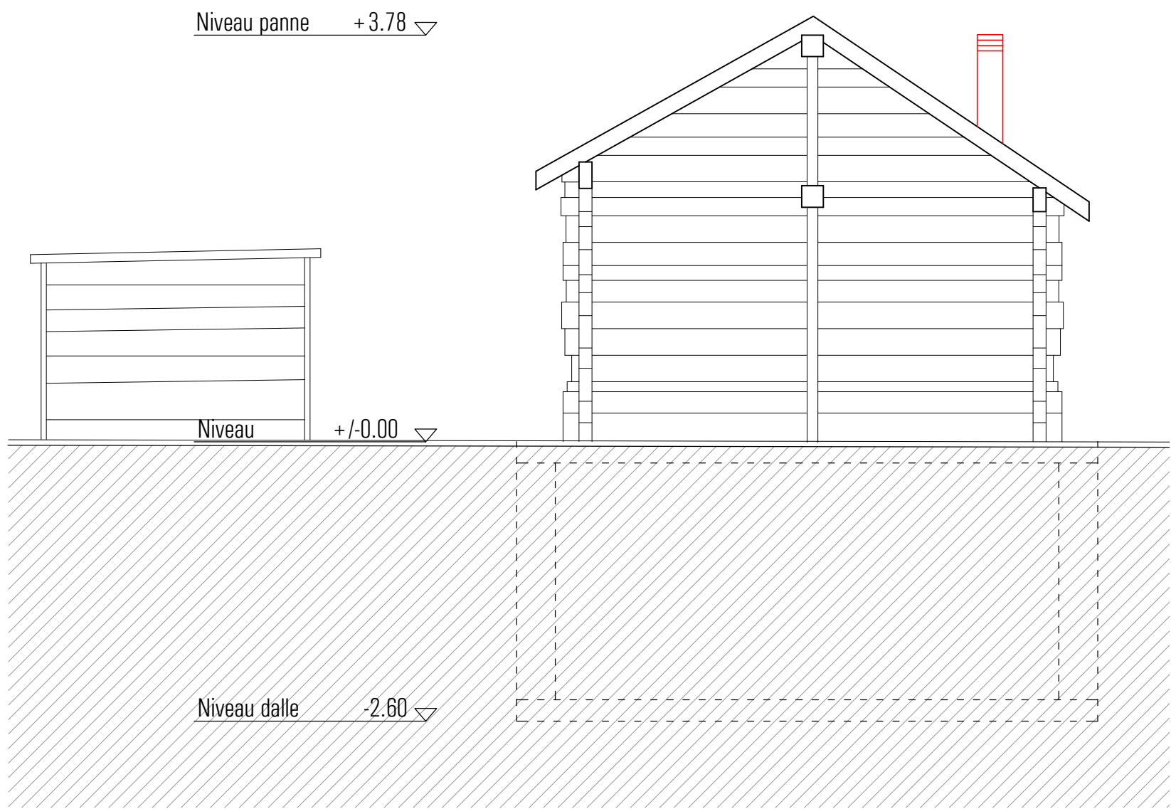
façade est
