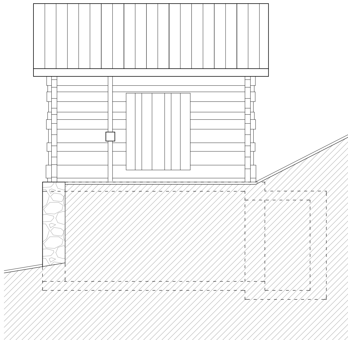
façade sud
